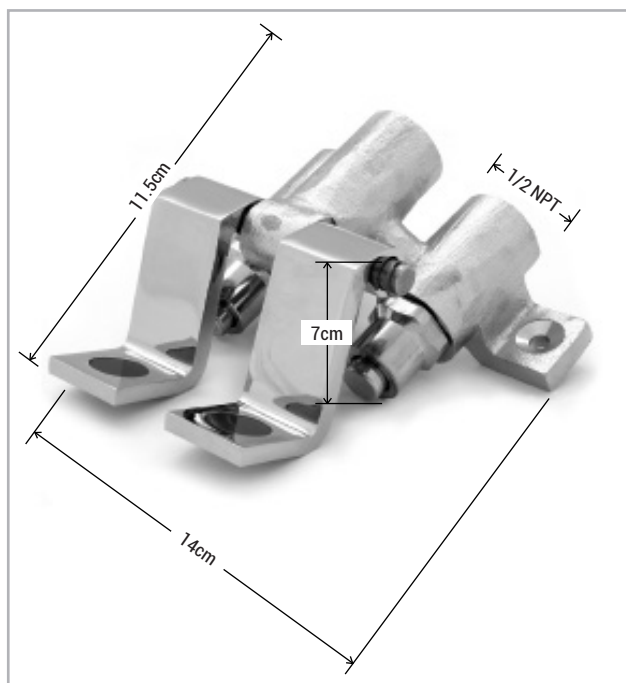
MEDIDAS DE LA LLAVE
